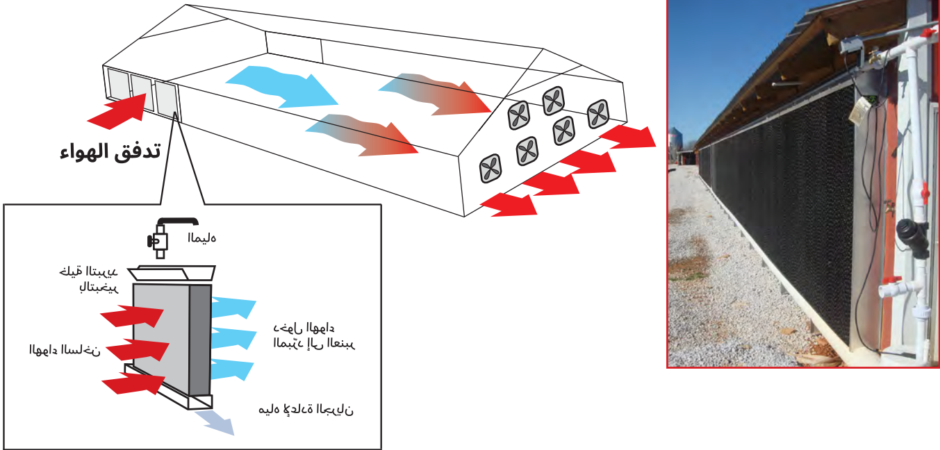
الصورة 19.6: تبريد الهواء بالخلايا مع التهوية النفقية.
