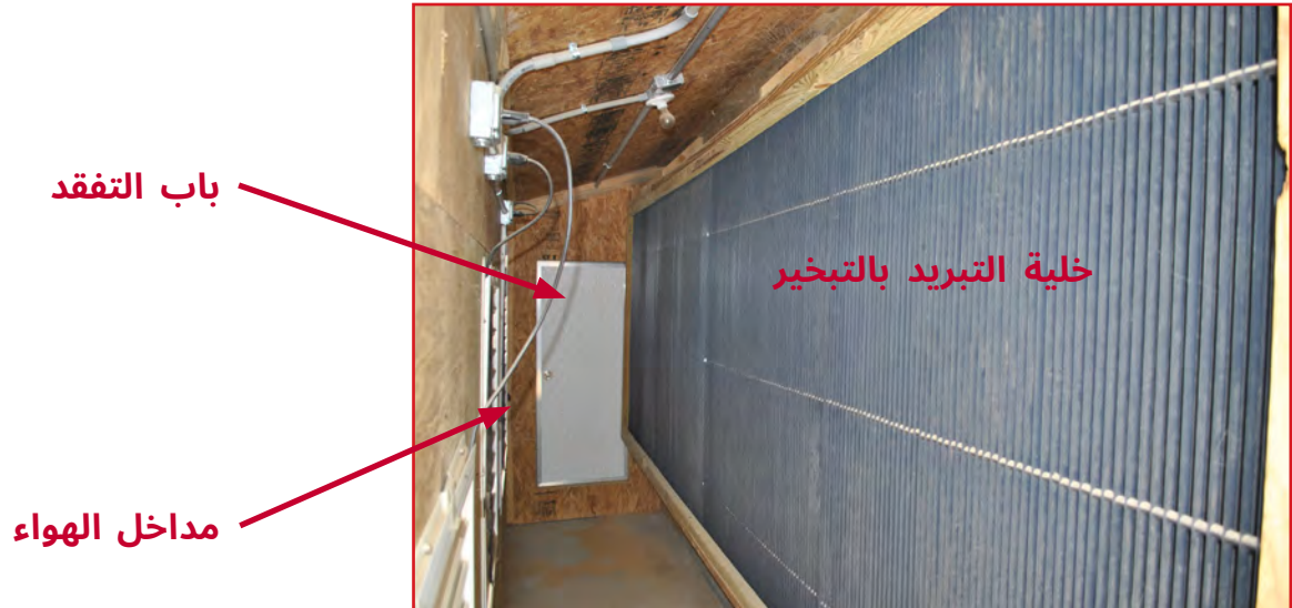
الصورة 20.6: مثال على خلايا تبريد مثبتة على الحائط الجانبي للعنبر في غرفة الدوجهاوس.
