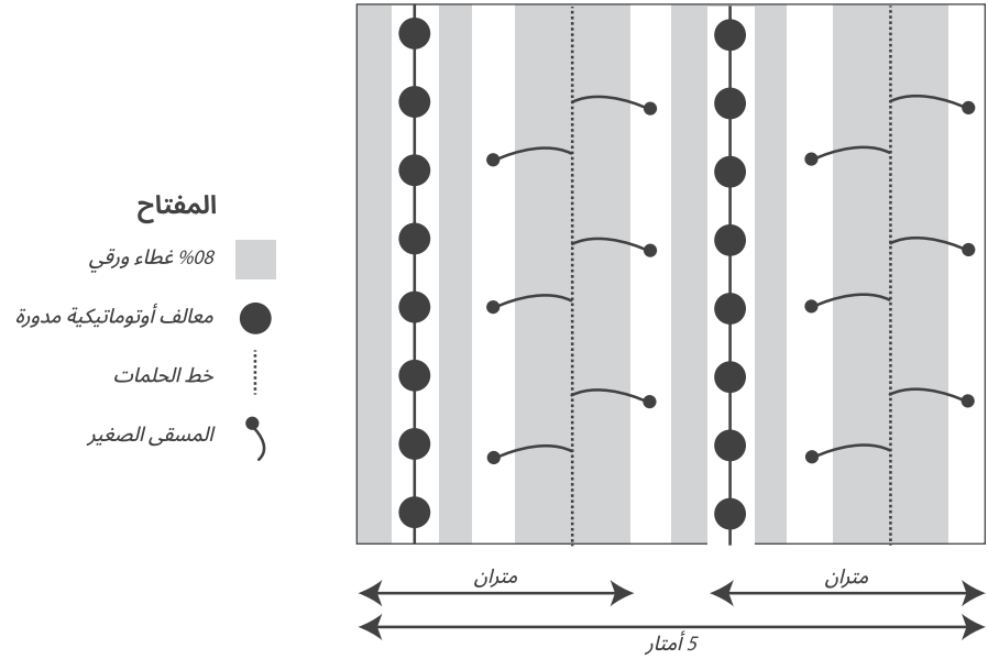
الشكل 7.2: المخطط المعتاد لنظام تحضين العنبر الكامل (1000 كتكوت).
