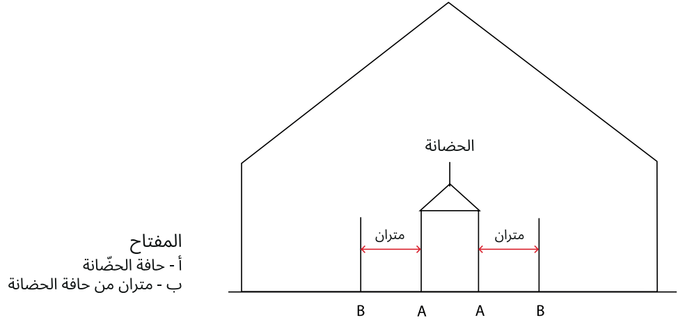
الشكل 5.2: التحضين الثابت - مناطق تدرّجات درجة الحرارة
