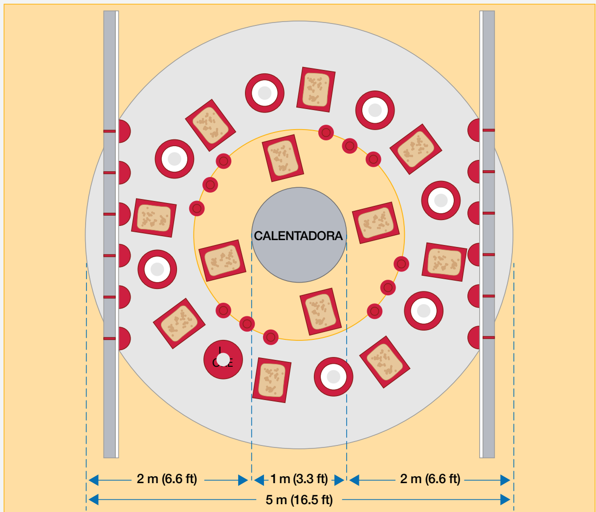
Figura 2.6 Ejemplo de una disposición típica de crianza por zonas (1000 pollos).
