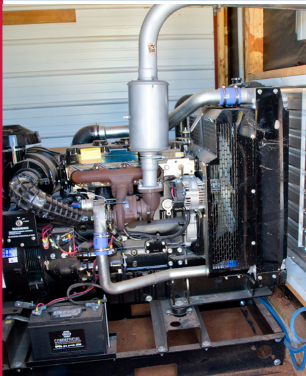
Figura 6.2 Ejemplo de un generador de reserva.
