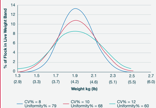
Figura 3.6 Efecto del CV % o la uniformidad % en las fajas de peso vivo en un lote de pollos de engorde sexados.
