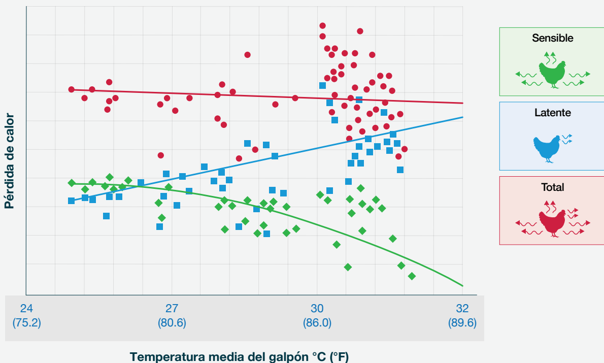
Figura 6.26 Pérdida de calor sensible y latente.
