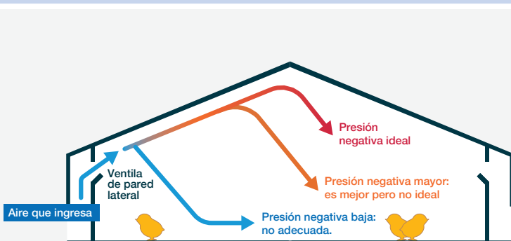
Figura 6.11 Uso de la presión negativa para controlar la velocidad del aire.
