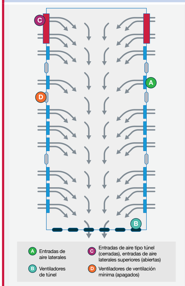
Figura 6.16 Movimiento típico del aire durante la ventilación de transición.
