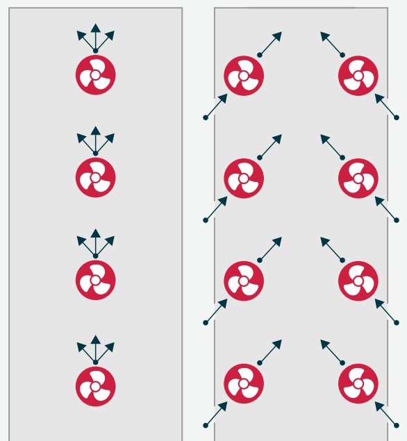
Figura 6.5 Disposición de los ventiladores de circulación: situados en el centro (izquierda) o cerca de la pared lateral/cortina (derecha).
