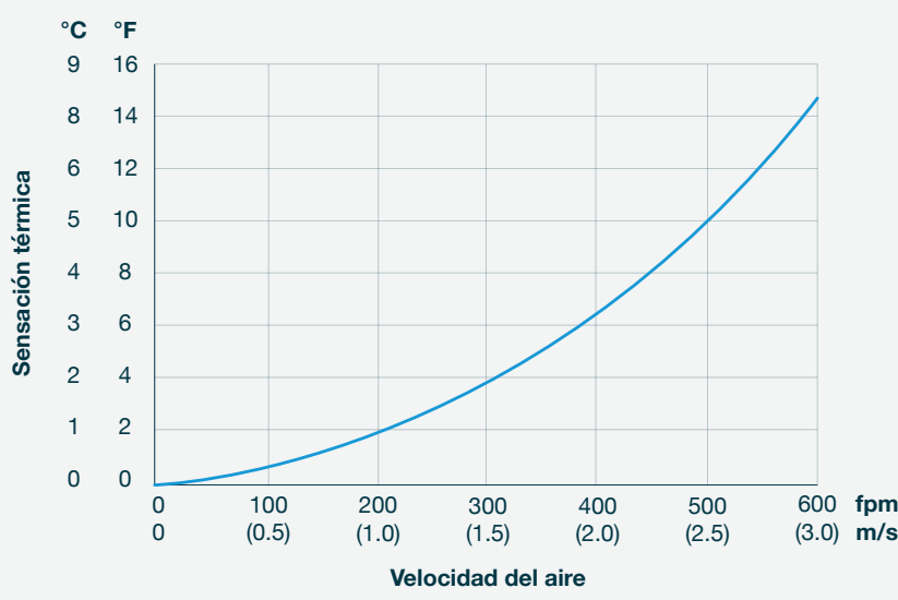
Figura 6.21 Efecto de enfriamiento teórico que siente un pollo de engorde de 3,5 kg (7,7 lb) a una temperatura del aire de 29,4 °C (85 °F).
