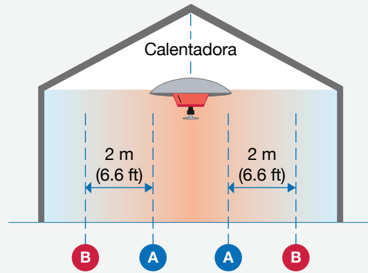
Figura 2.7 Gradientes de temperatura en la crianza por zonas.
