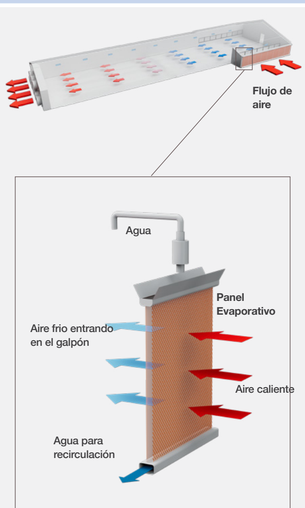
Figura 6.24 Enfriamiento por paneles con ventilación por túnel.
