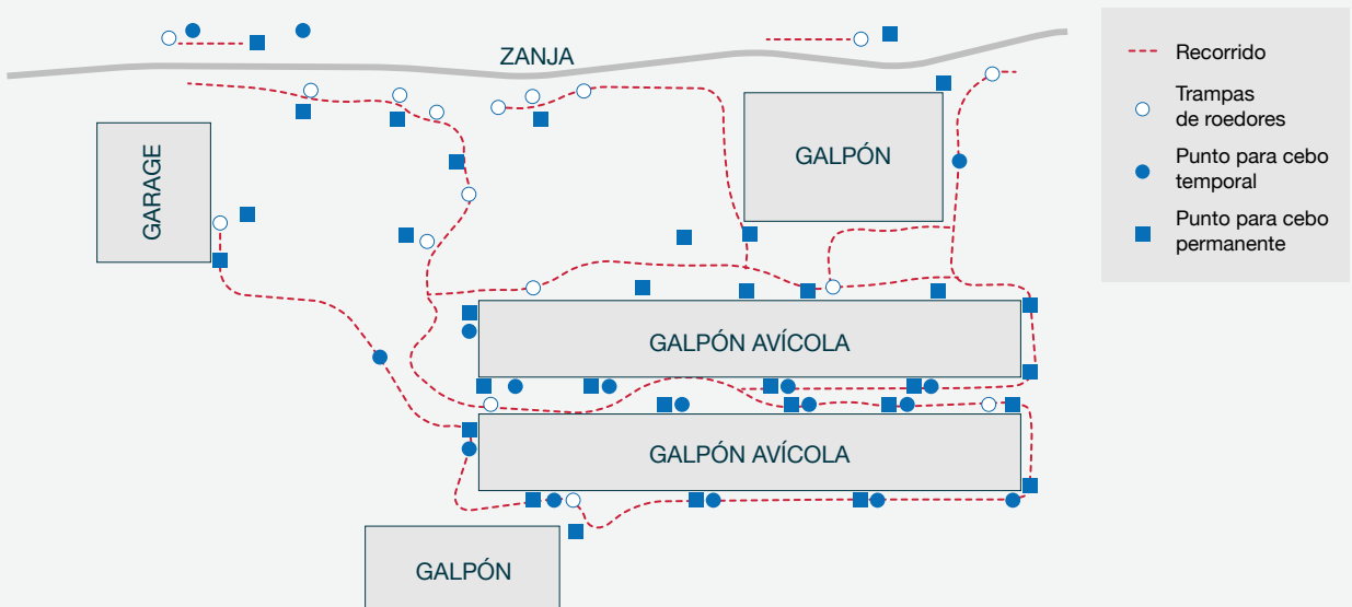
Figura 7.5 Ejemplo de un plan de cebos para roedores.
